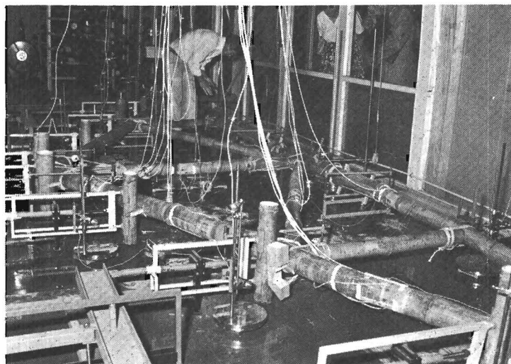
Een reuzenspan van bamboe (lengte acht meter) moest afgelopen weekeinde een forse belasting ondergaan. Pas bij een druk van 25 kg Newton begaf de span het. Dit alles in het kader van een promotie-onderzoek van ir. Jules Janssen (B) naar de constructiemogelijkheden in derde wereldlanden van bamboe. In de W-hal doet ir. Janssen al geruime tijd allerhande sterkteproeven met bamboe.
